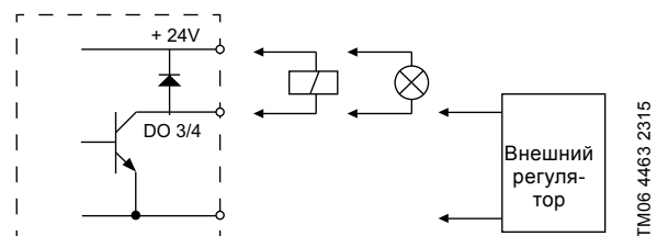
Рис. 69 Пример настраиваемых цифровых входов или выходов
