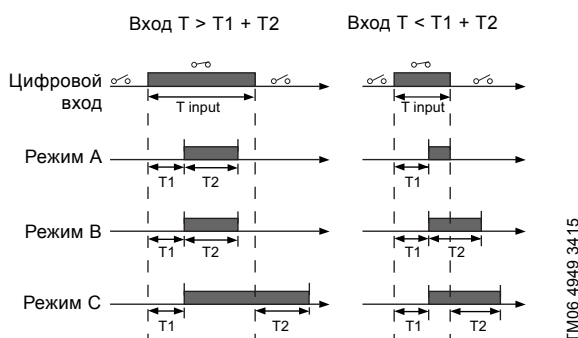
Рис. 68 Функция таймера длительности для цифровых входов
